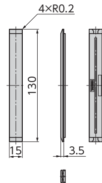
[FE-461-2-C] 連結ジョイント Joint
