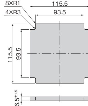
[FE-461-2-F-3] 不織布フィルター Non-woven filter
